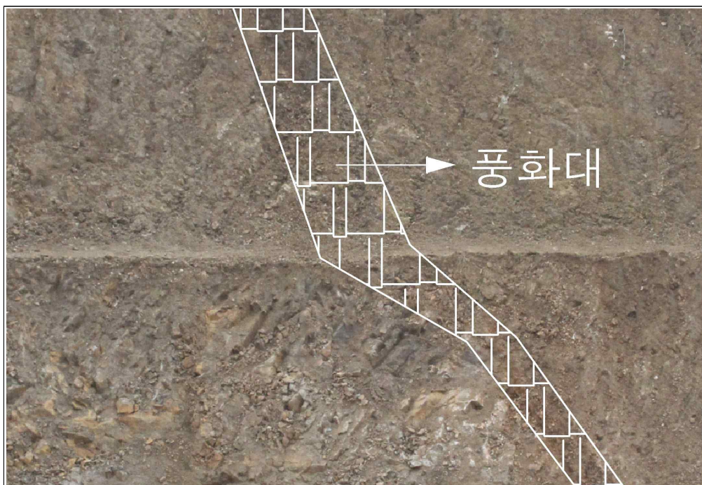
【그림 28】 D 영역 상세사진 (풍화대 발달)
