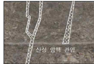
D영역 산성 암맥 관입
