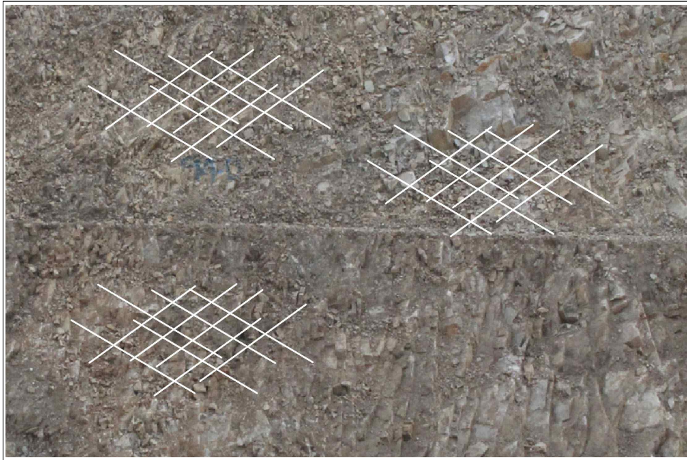
【그림 12】 A 영역 상세사진 (세편화된 암석)
