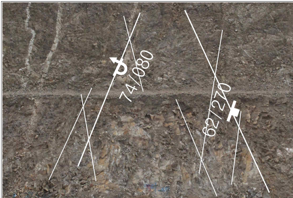
【그림 26】 D 영역에 발달한 불연속면
